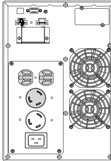
Рисунок 50. Модель PW9130G3000T-XL
